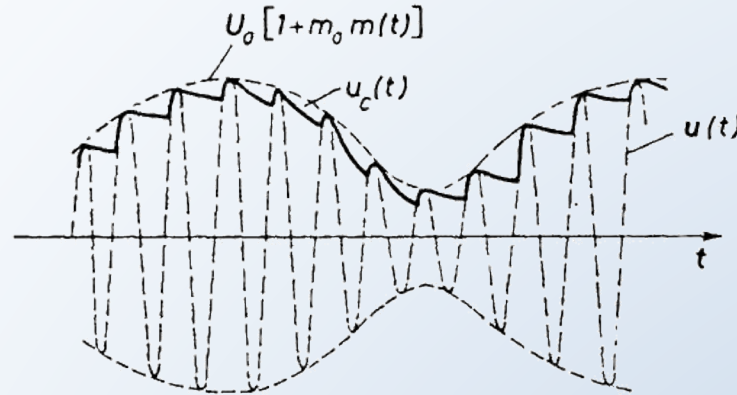
Slika: Amplitudski modulirani signal tipa KAM (isprekidano izvučena kriva) i detektovani napon u_c(t) (puno izvučena kriva)
